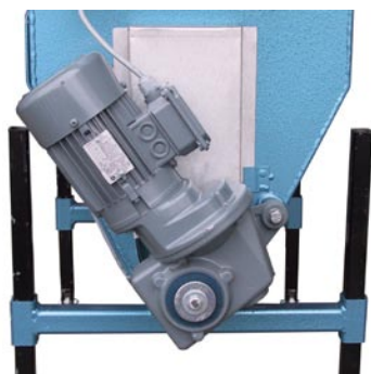
Kraftig motor, med ett vridmoment på hela 360 Nm, för bränsletransporten till förbränningsrummet
